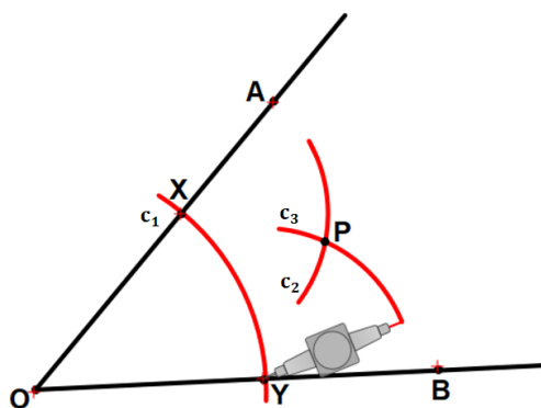
Figura 25 – Traçando a interseção entre os arcs c_2 e c_3
