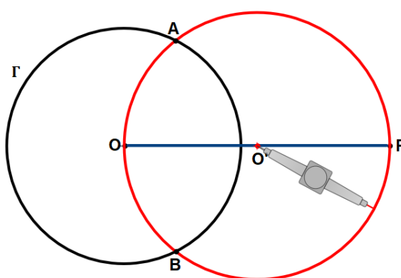
Figura 227 – Traçando o círculo de centro O' e raio \overline{O'O} = \overline{O'P}
