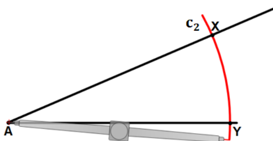
Figura 71 – Construção do arco de circunferência c_2
