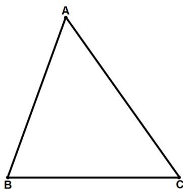
Figura 161 – Triângulo ABC
