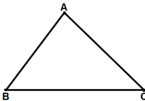
Figura 81 – Triângulo ABC
