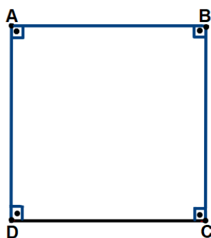
Figura 200 – Quadrado ABCD
