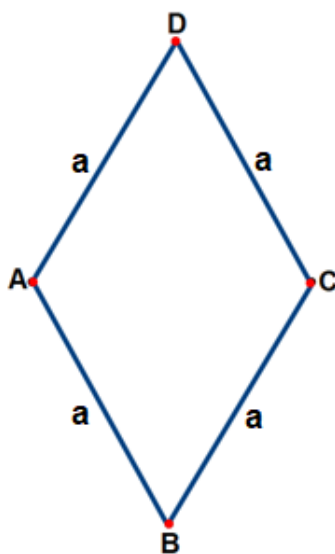
Figura 203 – Losango ABCD
